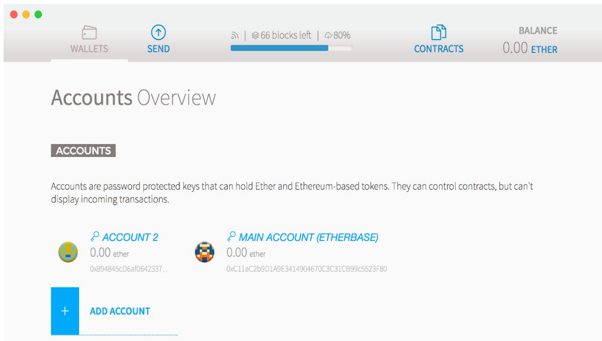
Mist browser
