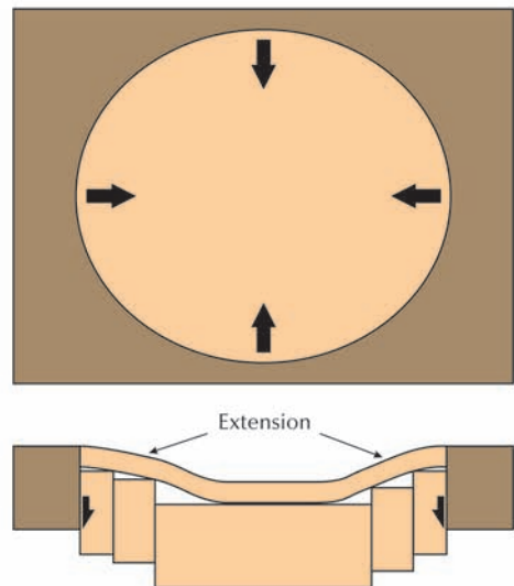
(d) Downsag
