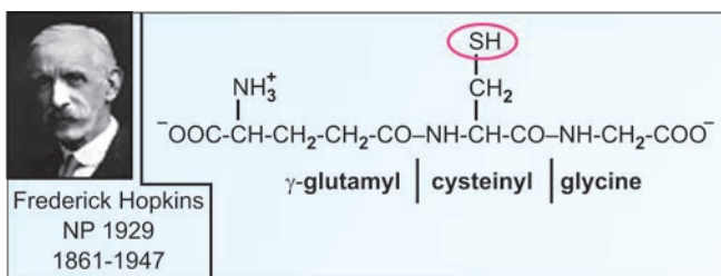
Fig. 15.19. Glutathione
