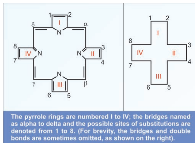
Fig. 21.2. Porphyrin ring
