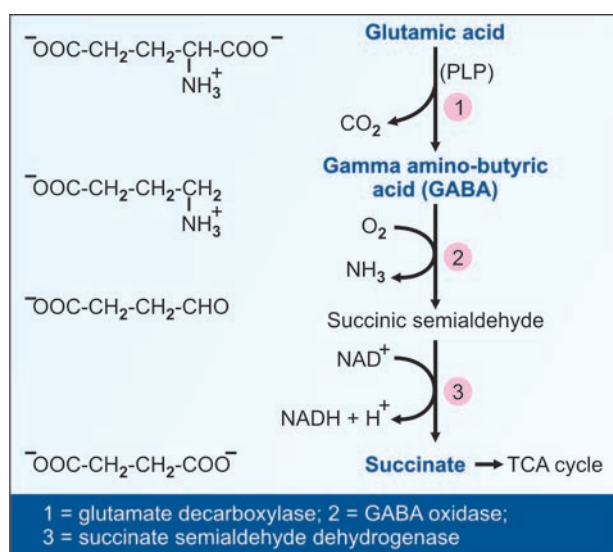
Fig. 16.2. GABA metabolism
