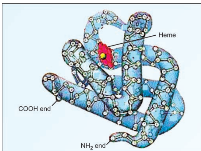
Fig. 22.14. Myoglobin chain
