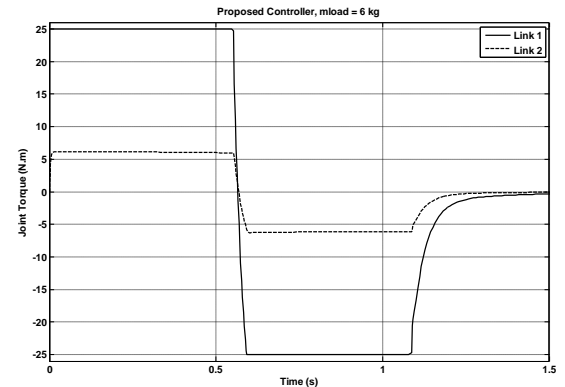
Fig 12. Motors torque.
